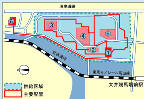
品川八潮団地地区熱供給システム図
