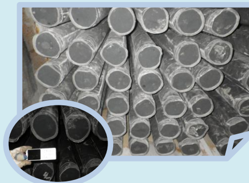
ろ過式集じん器内のろ布の写真です。 (1728本 直径約16cm×長さ6m)
